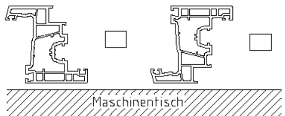
Profilaufgeseite Flügel
